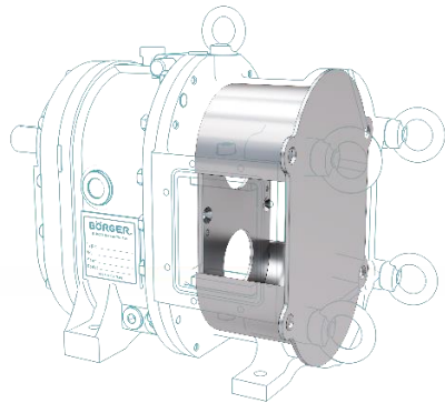
Udskiftelige foringer i pumpehus
